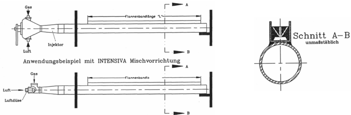
Langrohrbrenner Nr. 190
